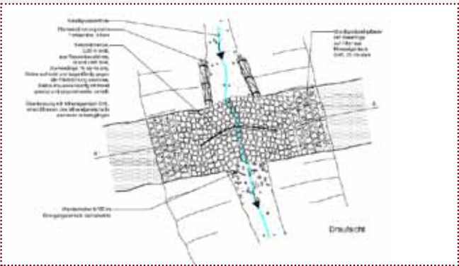
Konstruktionsdetail Setzsteinrampe als Furt Quelle: Ausführungsplanung, Planungsbüro Schubert, Radeberg
