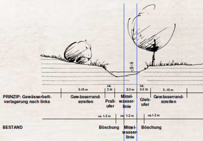
Aufwertung und leichte Gewässerbettverlagerung, Prallufer links Quelle: KÜHFUSS, LandschaftsArchitektur* Umweltplanung Dresden
